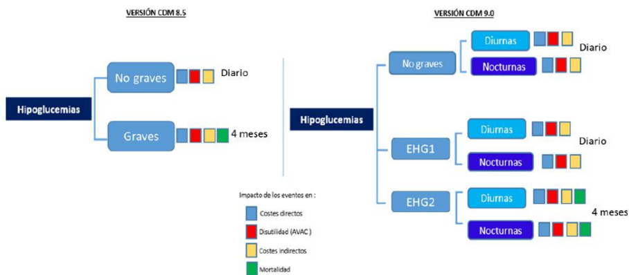
Figura 3. Modelo de hipoglucemias del CDM para DM1 y DM2
