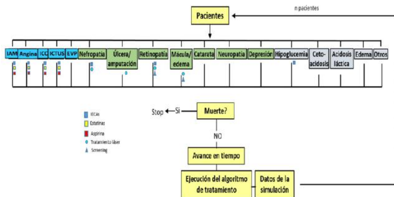
Figura 2. Estructura del CDM para DM1 y DM2
